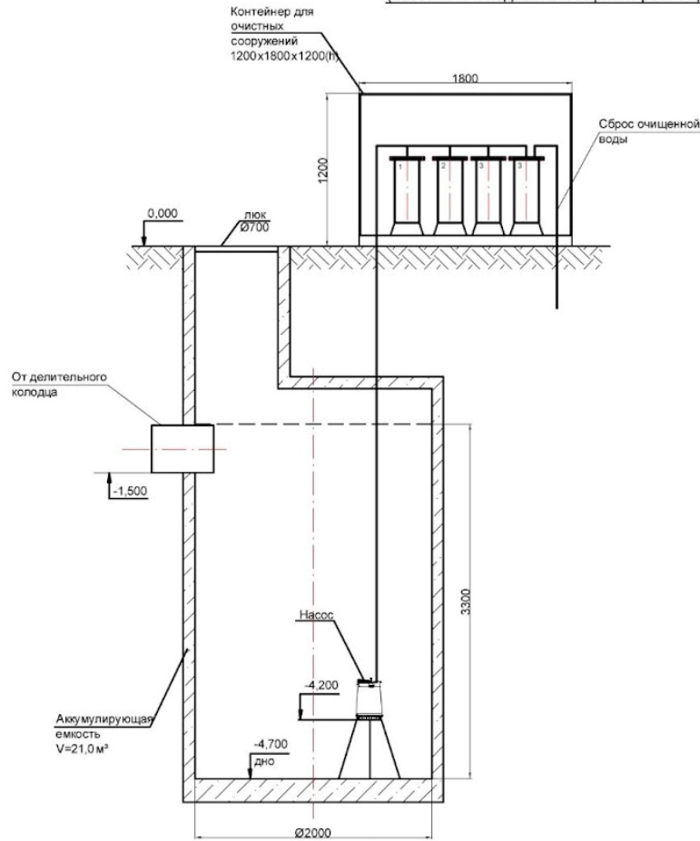
Принципиальная схема размещения оборудования очистных сооружений "НиВада" (наземный и подземный вариант размещения)
